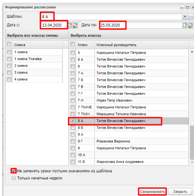
Рисунок 19 – Формирование расписания
